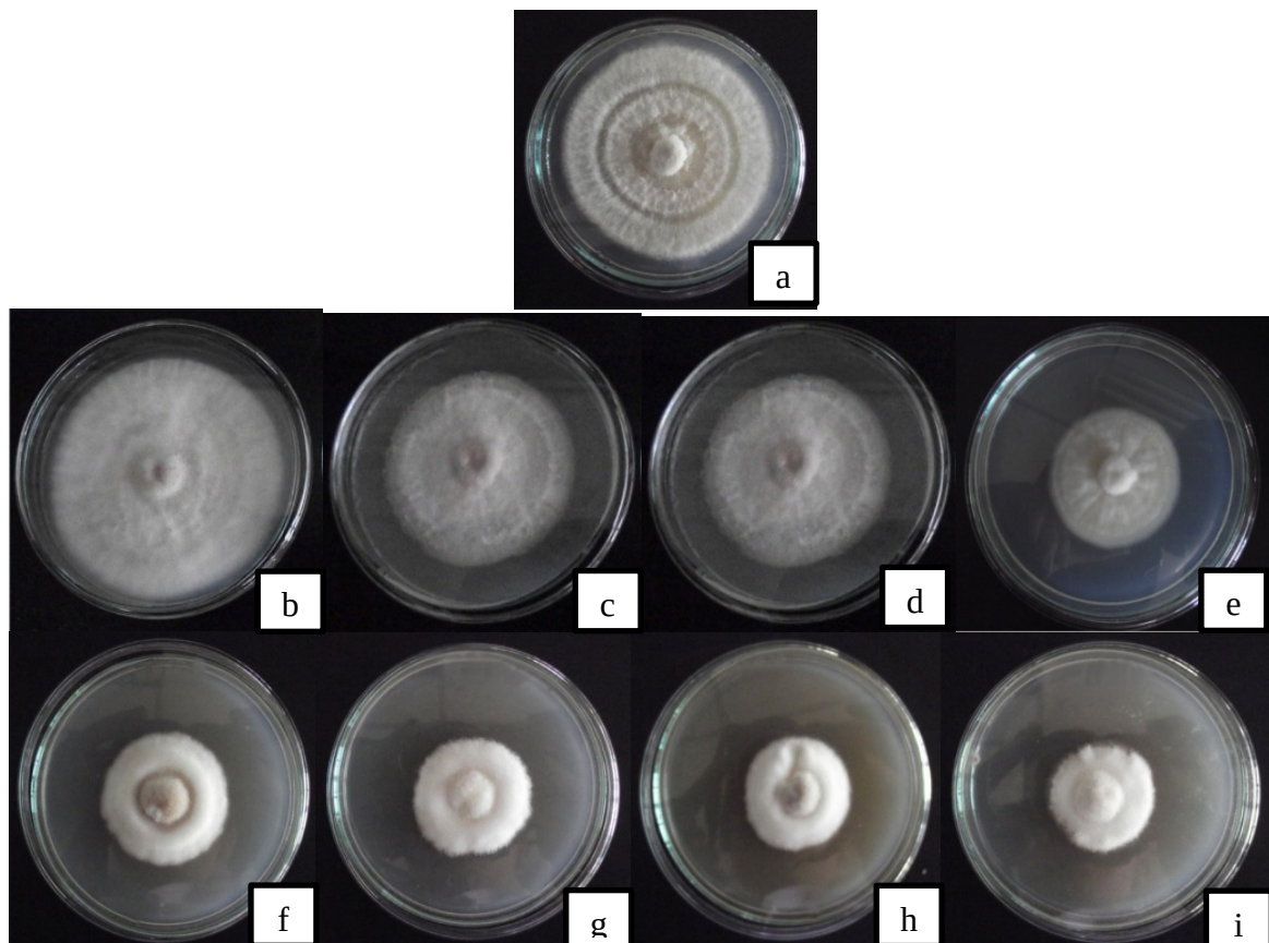
ภาพที่ 2 ผลของสารสกัดจากใบและผลของดิบมีประสิทธิภาพในการยับยั้งการเจริญของเส้นใยเชื้อรา C. gloeosporioides (a:ชุดควบคุม, b:ใบ 1250 ppm, c:ใบ 2500 ppm, d:ใบ 3750 ppm, e:ใบ 5000 ppm, f:ผล 1250 ppm, g:ผล 2500 ppm, h:ผล 3750 ppm, h:ผล 5000 ppm)
